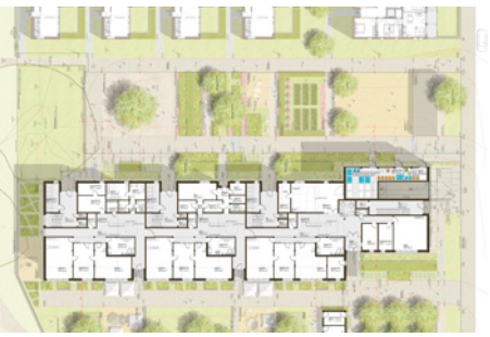
Grundriss EG mit Freianlagen
