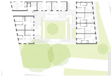
Grundriss OG
