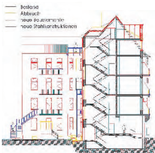
Die Hoffassade mit neuen Balkonen
